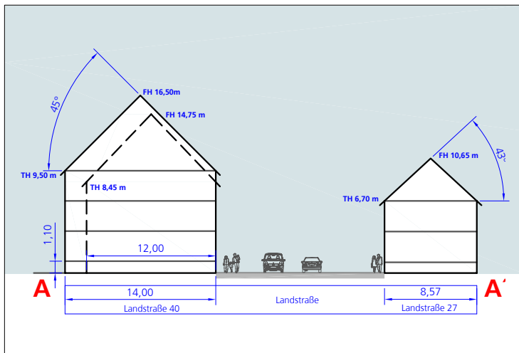
Straßenraumschnitt M 1:500
